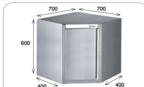
Armarios de pared angular 90°
