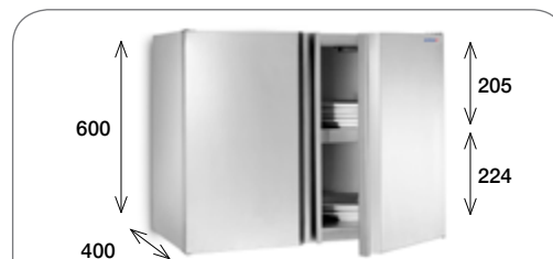
Armarios de pared puertas practicables
